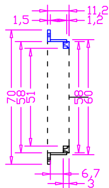
Leitschaufeln- Haltering
